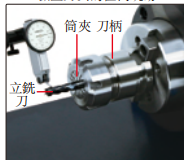
檢查刀具的徑向跳動
