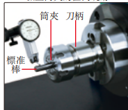
檢查刀具的徑向跳動
