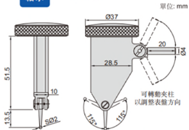
夾柱(標配)
