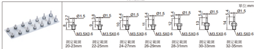
2223-62測頭(標配)
