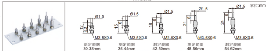
2223-153測頭(標配)
