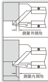
測量倒角尺寸
