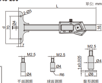
1148-P103(選配), 測量盲孔底部內溝槽的寬度
