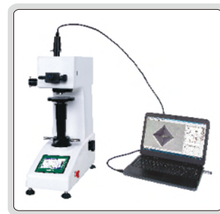
相機和測量系統(選配)
