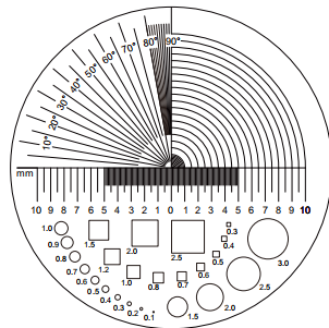
7527-D2底板刻綫 (0-5mm解析度0.1mm, 5-10mm解析度0.5mm)
